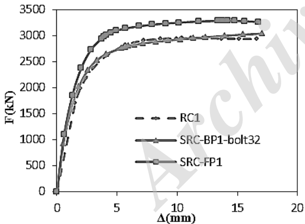
شکل ۹: مقایسه مقاومت دیوارهای برشی سه طبقه
