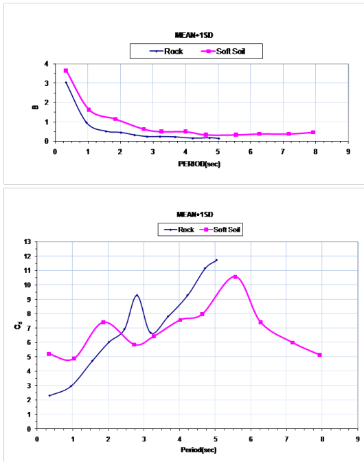
شکل ۷: ضرایب بزرگنمایی نیرو و تغییر مکان سیستم‌های لوله‌ای در تراز فوق میانگین برای تکیه گاه‌های صلب و انعطاف پذیر Fig. 7. The force and displacement amplification factors for the tubular systems at the average plus one Sigma level for rigid and flexible bases
