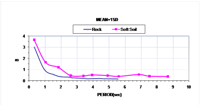
شکل ۹: ضرایب بزرگنمایی نیرو و تغییر مکان سیستم‌های مهاربند بازویی در تراز فوق میانگین برای تکیه گاه‌های صلب و انعطاف پذیر
