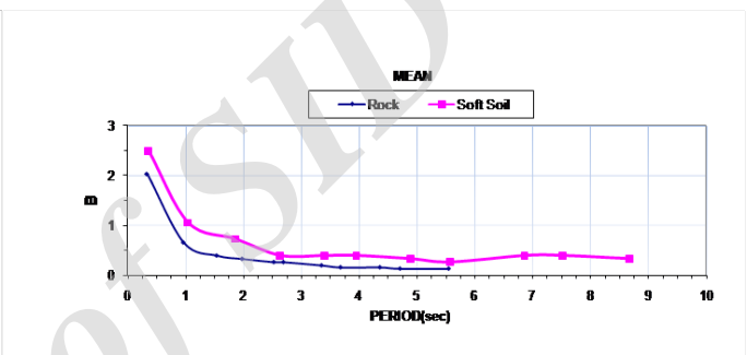
شکل ۱۰: ضرایب بزرگنمایی نیرو و تغییر مکان سیستم‌های مهاربند بازویی در تراز میانگین برای تکیه گاه‌های صلب و انعطاف پذیر
