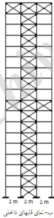
شکل ۳: پلان تیپ و نمای سازه مهار بازویی
