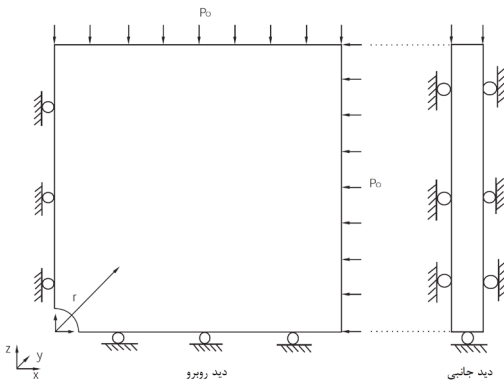
شکل ۴: شرایط مرزی در مدل ساخته شده در نرم افزار FLAC 3D
