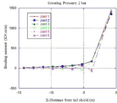
شکل ۲۴: روند تغییرات ممان خمشی در درزه‌های طولی سگمتی‌ها بر اساس فاصله از انتهای سپر برای حالت تزریق با فشار ۲ بار
