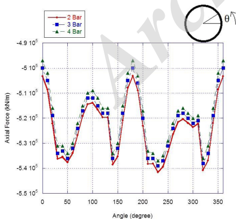
شکل ۲۶: نیروی محوری وارد بر آخرین مقطع پوشش یکپارچه (مجاور انتهای سپر) تحت تزریق با فشارهای مختلف
