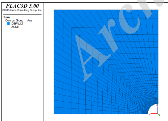
شکل ۵: شبکه بندی مدل در نرم افزار FLAC 3D
