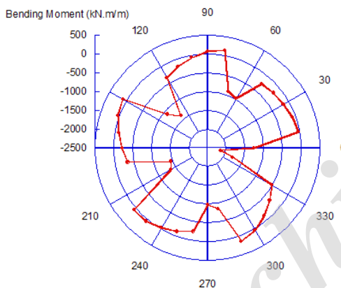
شکل ۱۹: ممان خمشی وارد بر آخرین حلقه سگمتنی (مجاور انتهای سپر) تحت تزریق با فشار ۴ بار
