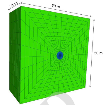
شکل ۸: ابعاد مدل تونل سبزکوه در نرم‌افزار FLAC 3D
