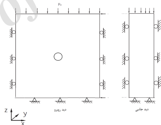
شکل ۹: شرایط اولیه و مرزی تونل سبزکوه در نرم‌افزار FLAC 3D
