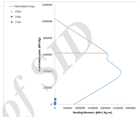
شکل ۲۷: نمودار اندرکنش نیروی محوری - ممان خمشی جهت کنترل پایداری سگمتی‌ها تحت فشار تزریق ۲، ۳ و ۴ بار
