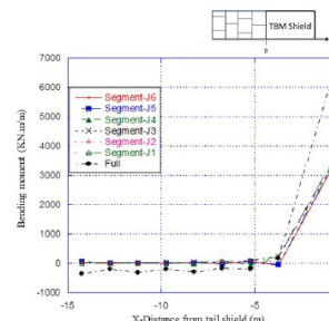
شکل ۱۴: ممان خمشی وارد بر پوشش سگمتی و پوشش یکپارچه در محل درزه‌ها بر اساس فاصله از انتهای سپر
