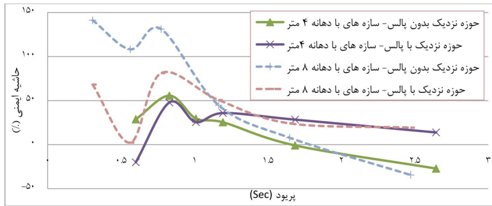
شکل ۱۳: منحنی‌های تغییرات «حاشیه ایمنی» بر حسب پریود مود اول سازه‌ها در گروه‌های عملکردی ۱۱۱-۱۱۲ (سازه‌های با دهانه ۴ متر) و ۱۲۱-۱۲۲ (سازه‌های با دهانه ۸ متر) تحت تاثیر دسته رکوردهای حوزه نزدیک بدون پالس و با پالس
