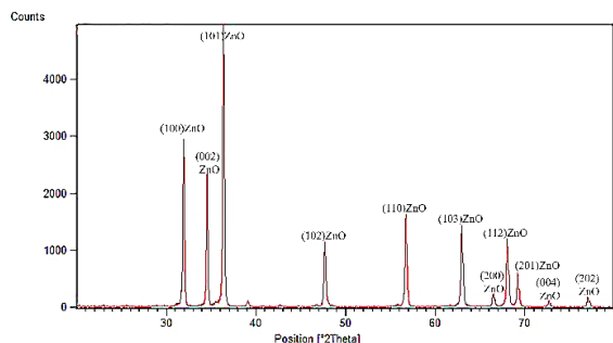
شکل ۶: نمودار پراش اشعه ایکس نانو اکسیدروی
