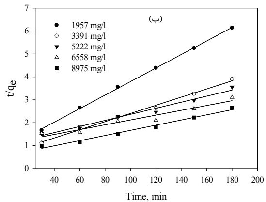
شکل ۷: نمودار سینتیکی شبه مرتبه اول (الف) و شبه مرتبه دوم (ب) (دما ۲۵ درجه سانتی گراد، pH= ۲، سرعت همزدن ۲۰۰ rpm، دوز جذب ۵۰ گرم بر لیتر)
