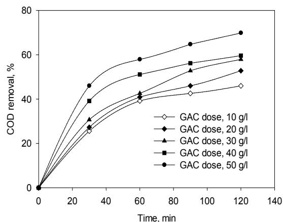
شکل ۱: روند حذف COD با مقادیر متفاوت طی زمان Fig. 1. COD removal trend in different GAC doses by time
