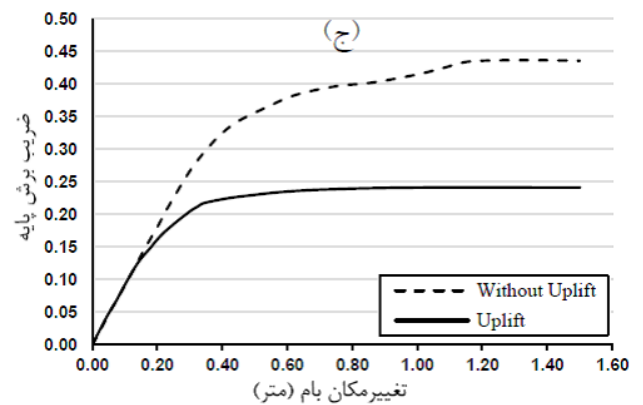
شکل ۲: نمودار برش پایه برحسب تغییر مکان بام برای الف) قاب خمشی m5x2، ب) سیستم دوگانه b5x2، ج) قاب خمشی U m10x2؛ با برکنش، W/U بدون برکنش)
