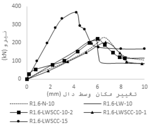
شکل ۵: منحنی‌های بار-تغییر مکان برای دال‌های با نسبت آرماتور ۱/۶
