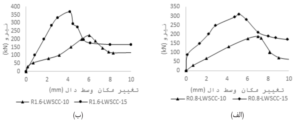
شکل ۷: تأثیر افزایش ضخامت دال بر ظرفیت برش دوطرفه دال‌های خودمترکم شونده سبک
