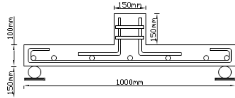
شکل ۱: مشخصات هندسی نمونه‌های آزمایشگاهی
