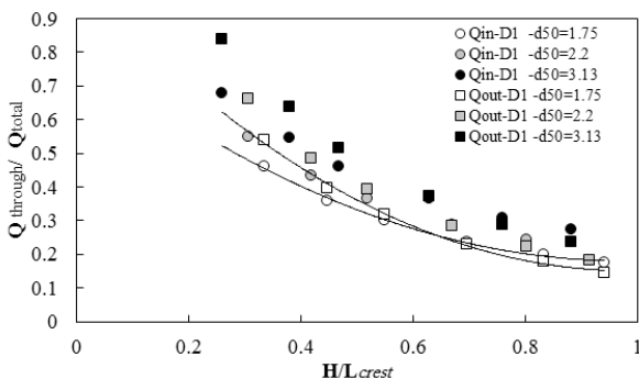
شکل ۱۲: مقایسه دبی ورودی از سطح جلو و دبی خروجی از انتهای سرریز متخلخل برای سرریز با شیب پایین دست ۴۵ درجه
