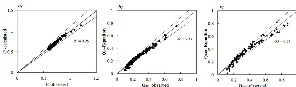
شکل ۱۵: مقایسه مقادیر محاسباتی و مشاهده شده برای (a) ضریب دبی (b) دبی ورودی از بالادست
