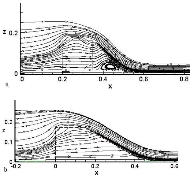
شکل ۱۳: الگوی جریان اطراف سرریزهای متخلخل گابیونی (الف) مربعی (ب) ذوزنقه‌ای با شیب پایین دست
