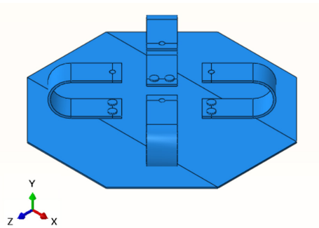
شکل ۱۱: مدل چیدمان ۴ تایی میراگر U شکل
