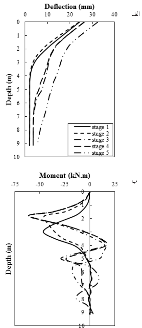
شکل ۵: نتایج حاصل از مدل عددی در مراحل مختلف الف) جابجایی افقی دیوار ب) لنگر خمشی دیوار
