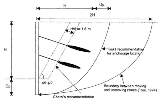
شکل ۹: مکان طول گیردار مهار پیشنهاد شده توسط [۲۴]، [۲۵]
