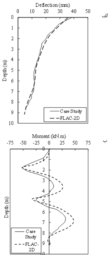
شکل ۶: مقایسه نتایج مدلسازی با مطالعه موردی و صحت‌سنجی الف) جابجایی افقی دیوار ب) لنگر خمشی دیوار
