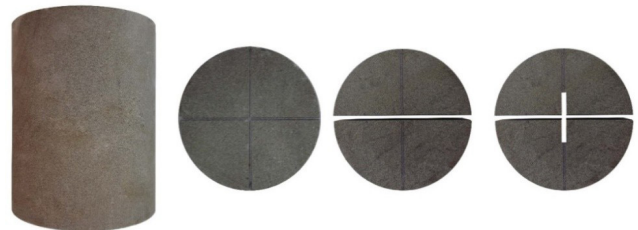
شکل ۴: مراحل آماده‌سازی نمونه (Semi-Circular Specimen) SCB
