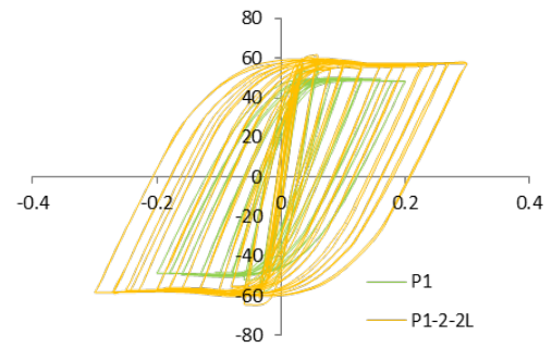
شکل ۱۷: مقایسه منحنی پوش بار-جابجایی
