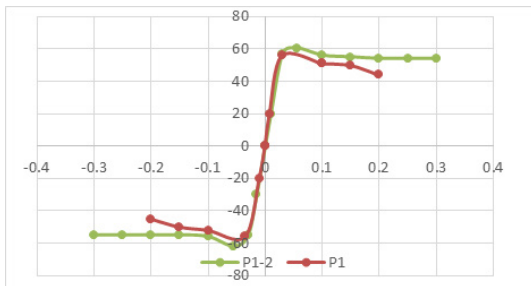
شکل ۱۶: مقایسه منحنی هیستریسیس بار-جابجایی
