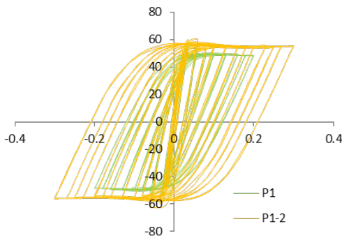
شکل ۱۵: مقایسه منحنی هیستریسیس بار-جابجایی
