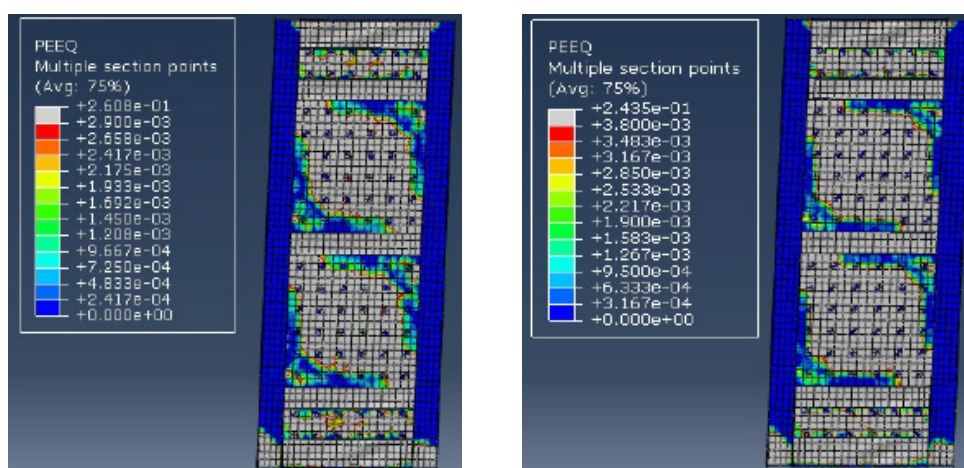
شکل ۹. توزیع کرنش های اصلی در رویه بتنی در تغییرمکان جانبی برابر ۲۵۰ mm. (الف) بتن با مقاومت ۳۵ و (ب) با مقاومت ۱۴ مگاپاسکال
