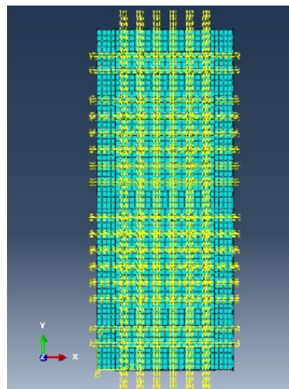
شکل ۲. مدل اجزا محدود دیوار برشی آزمایشگاهی
