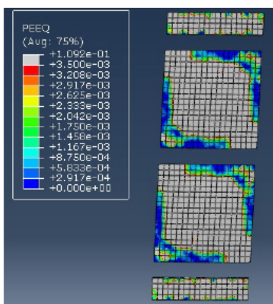
شکل ۷. توزیع کرنش‌های اصلی در رویه بتنی
