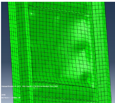
شکل ۱۲. نمای دیوار در تغییرمکان جانبی برابر با ۵۰ میلی و وقتی فاصله برش گیرها ۷۵۰ میلی می باشد
