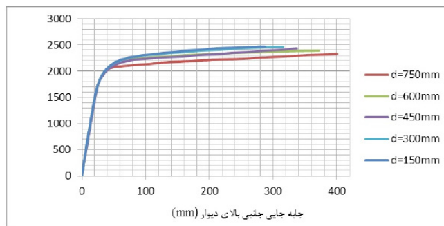
شکل ۱۰. برش پایه بر حسب جابه جایی جانبی بالای دیوار برای فواصل مختلف برش گیرها
