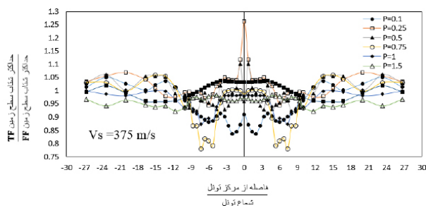
شکل ۵. بزرگنمایی شتاب حداکثر سطح زمین در خاک تیپ III-II (عمق تونل h/a=2 )
