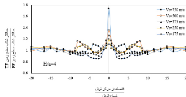
شکل ۱۳. بزرگنمایی شتاب سطح زمین در انواع خاک در تونلی به عمق H/a=4
