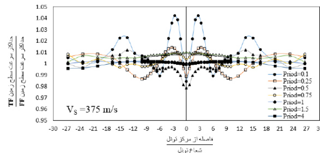
شکل ۶. بزرگنمایی سرعت حداکثر سطح زمین در خاک تیپ III-II (عمق تونل h/a=2 )
