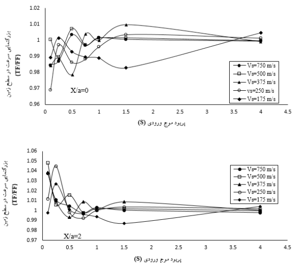
شکل ۹. بزرگنمایی سرعت سطح زمین در پرپودهای موج ورودی X/a=2 و X/a=0 تا ۴ ثانیه در فاصله X/a=0 و X/a=2
