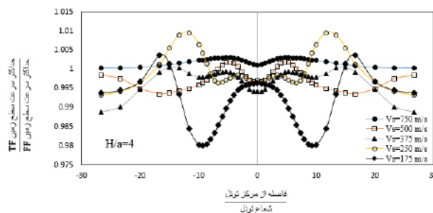
شکل ۱۴. بزرگنمایی سرعت سطح زمین در انواع خاک در حضور تونلی به عمق H/a=4
