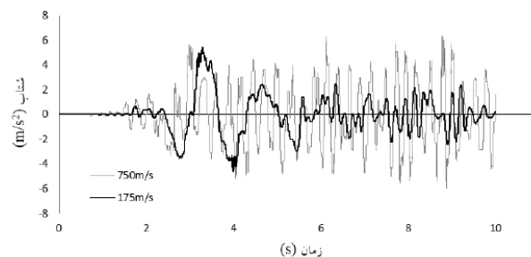
شکل ۱۲. تاریخچه شتاب سطح زمین در شرایط حضور تونل برای دو نوع خاک تیپ II-I و تیپ IV-III
