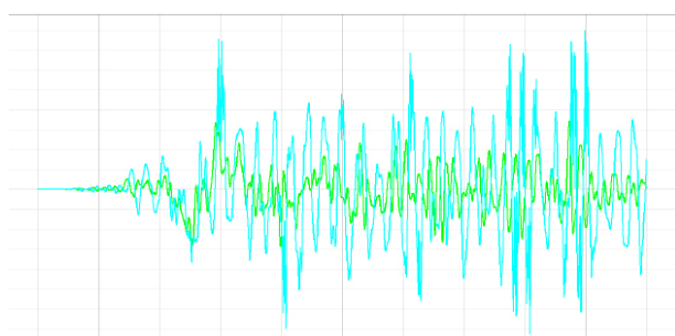
شکل ۱۰. شتاب‌نگاشت اعمال شده به کف مدل و برداشت شده در سطح زمین در خاک تپ II-I و تونل به عمق H/a=4
