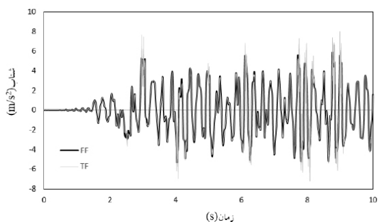
شکل ۱۱. شتاب‌نگاشت‌های سطح زمین بدون تونل و با حضور تونل
