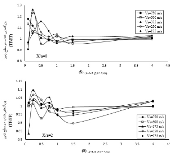
شکل ۸. بزرگنمایی شتاب سطح زمین در پرپودهای موج ورودی X/a=2 و X/a=0 تا ۴ ثانیه در فاصله X/a=0 و X/a=2
