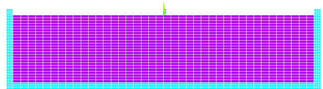
شکل ۲. نمای کلی از مخزن دوبعدی شبکه بندی شده
