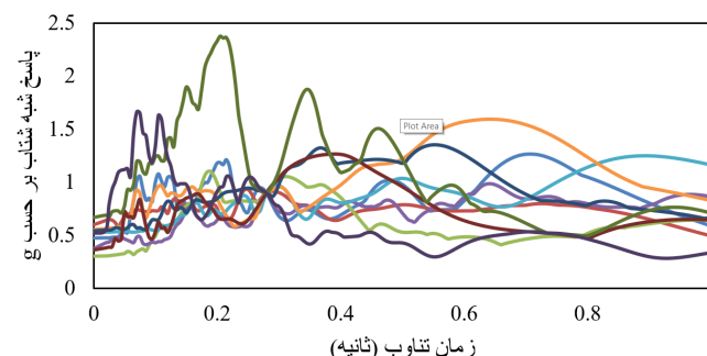
شکل ۷. طیف های پاسخ مقیاس شده زلزله های حوزه دور برای مخزن ۴۰×۹ Fig 7. Scaled response spectrum of far-field earthquakes for case 40 x9
