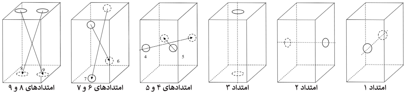
شکل ۳. امتدادهای در نظر گرفته شده برای انتشار امواج صوتی در نمونه‌های سنگ گرانیتی Fig3. Orientations considered for waves propagation in granitic rocks samples
