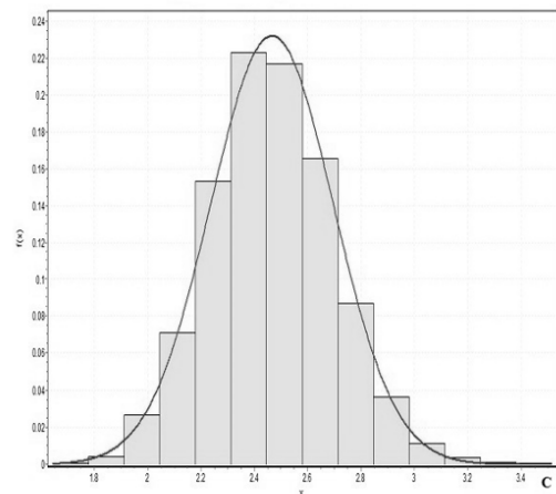
شکل ۹ توزیع حاشیه ای پارامتر C Marginal Distribution of T C \sim \text{Normal} (2/5179, 0/0490)
