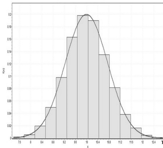
شکل ۸ توزیع حاشیه ای پارامتر T Marginal Distribution of \alpha T \sim \text{Normal} (10/2865, 0/4395)
