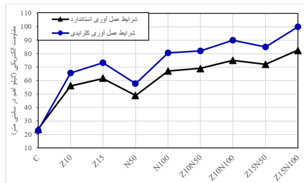
شکل ۱۱. نمودار مقاومت الکتریکی نمونه‌ها در شرایط عمل آوری استاندارد و کلرایدی در سن ۹۰ روز Fig11. The electrical resistance values under Standard and chloride curing condition at the age of 90 days
