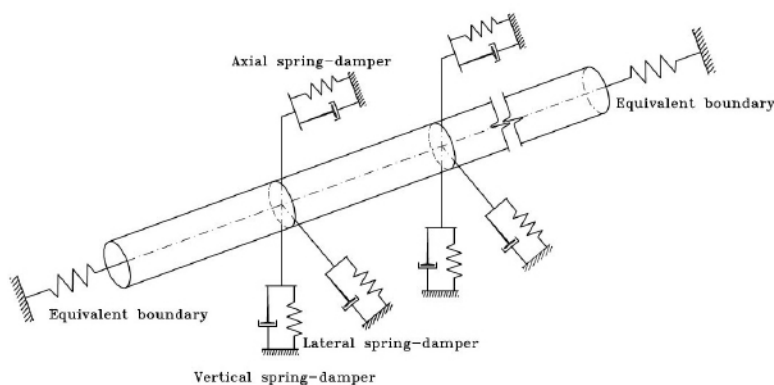
شکل ۱. تصویر شماتیک سیستم خاک-لوله [۱۴]
