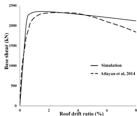
شکل ۶. مقایسه منحنی ظرفیت مدل قاب پنج طبقه مرکب 3-HBRB در مطالعه حاضر با نتایج مرجع [۱۴]
