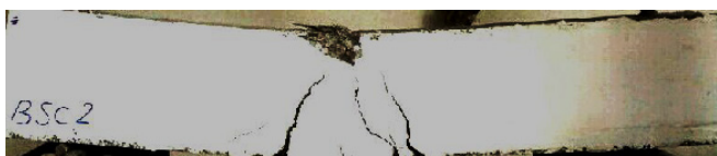
شکل ۲۴. وضعیت انتشار ترک در نمونه‌ی BSC2 پس از پایان بارگذاری-باربرداری
