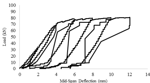
شکل ۲۱. نمودار بارگذاری-باربرداری نمونه‌ی BSC2
