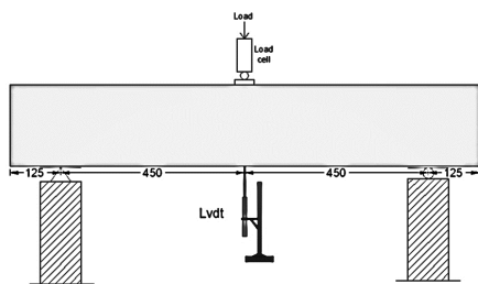
شکل ۵. پیکربندی آزمایش
