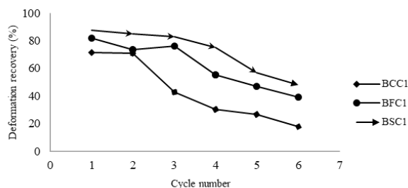
شکل ۲۵. نمودار مقایسه‌ای قابلیت بازیابی تغییر شکل تیرهای BCC1، BFC1 و BSC1
