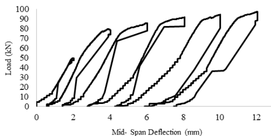
شکل ۲۰. نمودار بارگذاری-باربرداری نمونه‌ی BFC2
