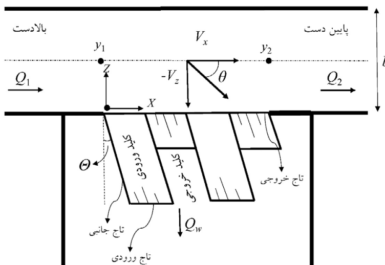
شکل ۴. طرح شماتیک از مشخصات هندسی سرریز و کانال اصلی
