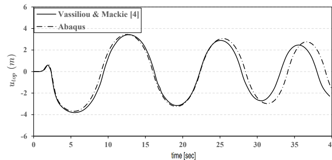
شکل ۹. تغییر مکان نوک بلوک انعطاف پذیر شماره ۲ Fig. 9. Top deflection of flexible Block 2
