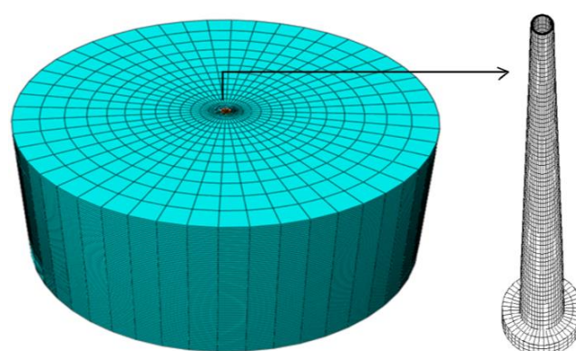
شکل ۶. مدل المان محدود برج آبگیر و مخزن سد بریونز در حالت مستغرق
