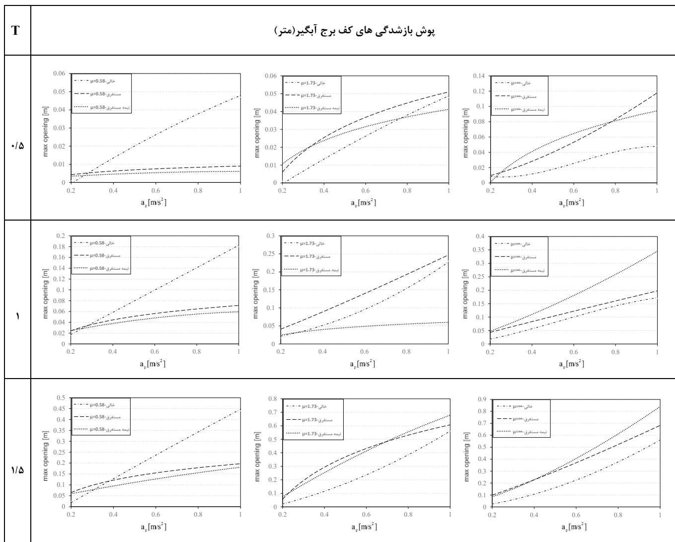
شکل ۱۶. پوش بازشدگی های کف برج آنگیر در حالات مختلف تحت سه پالس با زمان تناوب ۰/۵، ۱ و ۱/۵ ثانیه Fig. 16. Envelope of tower's base opening in different conditions under pulses with periods of 0.5, 1.0 and 1.5 sec
