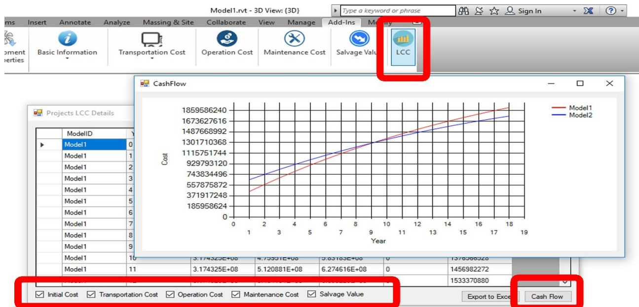
شکل ۱۲. نمای کلی انتخاب اجزای هزینه‌های چرخه عمر نمودار جریان نقدینگی در ابزار توسعه یافته Fig. 12. Overview of life cycle cost selection components of cash flow chart in the developed tool box
