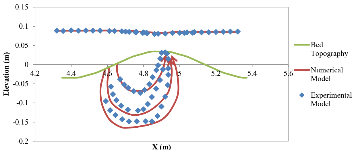
شکل ۵: خطوط جریان هایپریک مشاهده‌ای و شبیه‌سازی شده Fig. 5. Observed and simulated hyporheic path lines
