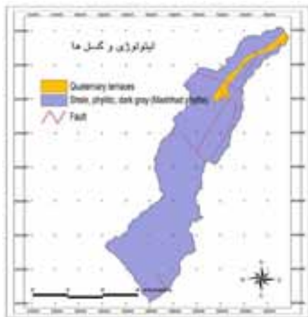
شکل (۵): لیتولوژی و گسل‌ها**
