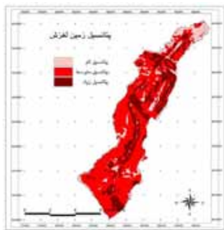
شکل (۷): پتانسیل زمین لغزش**
