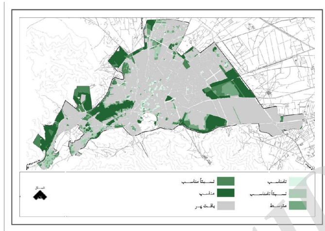
نقشه ۱۳: تحلیل مناسبت کاربری زمین برای استقرار کاربری تفریحی و سبز شهری
