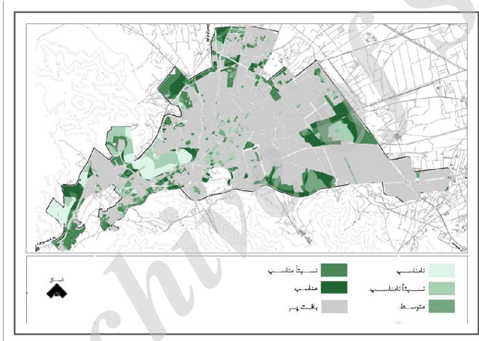
نقشه ۱۲: تحلیل مناسبت کاربری زمین برای استقرار کاربری تفریحی و سبز ناحیه‌ای
