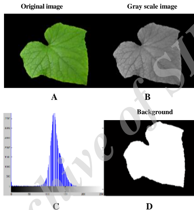
شکل ۴- الف: فضای RGB، ب: فضای Gray scale، ج: هیستوگرام تصویر Gray scale، د: جداسازی برگ از پس زمینه (اصلی) Figure 4. A: RGB space, B: Gray scale space, C: Histogram of the image gray scale, D: Leaf separating of background (Original)
