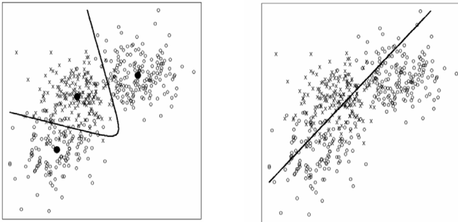
شکل ۱: کران تصمیم بین دو کلاس سمت چپ MDA سمت راست LDA
