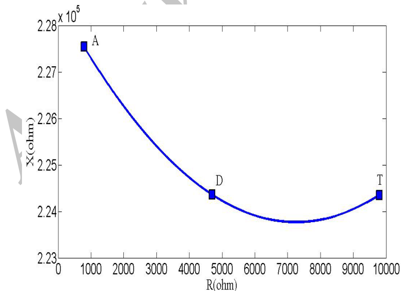
شکل ۱۸. منحنی تغییرات راکتانس پروب بر حسب مقاومت پروب در بازرسی لوله فولاد زنگ‌نزن برای موقعیت‌های مختلف
