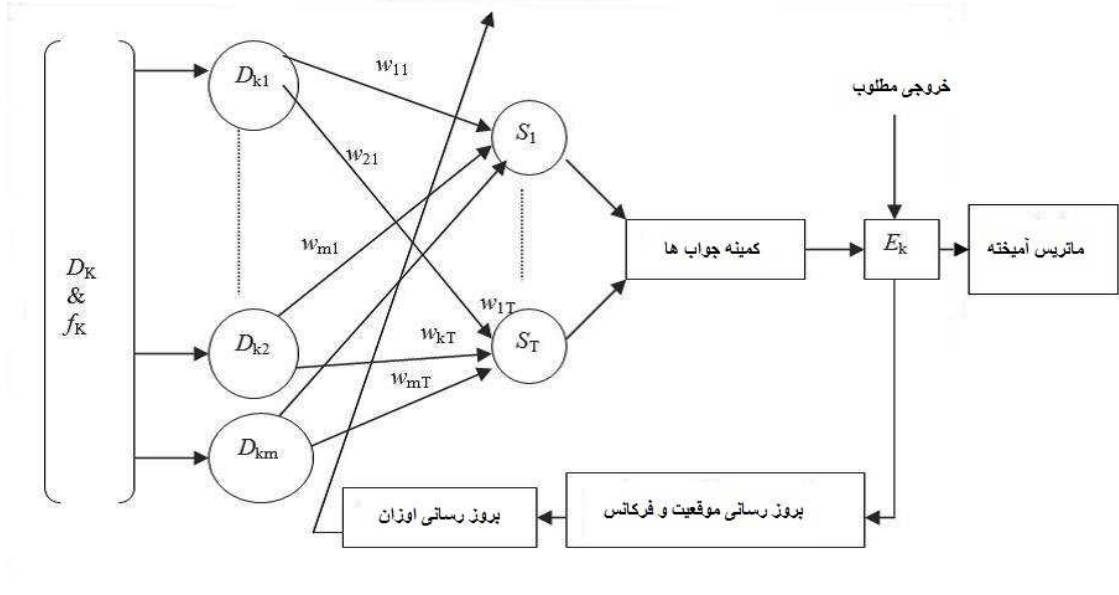
شکل ۴. الگوریتم بت
