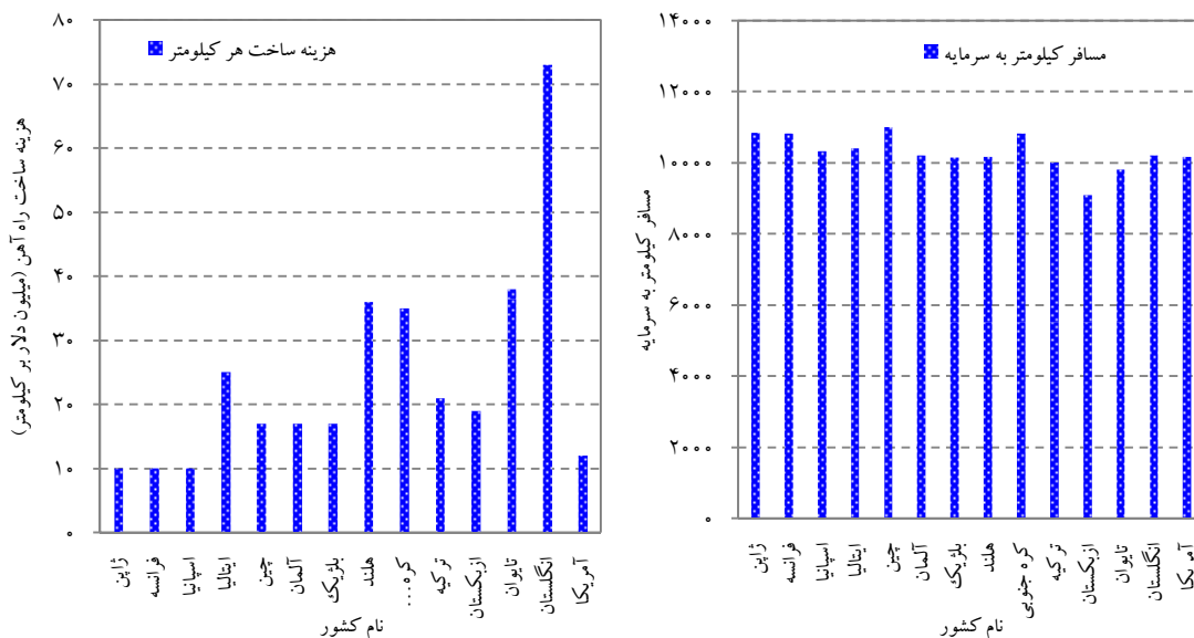
شکل ۱۱. راست: شاخص مسافر-کیلومتر به سرمایه، چپ: شاخص هزینه ساخت راه‌آهن سریع‌السیر در هر کیلومتر
