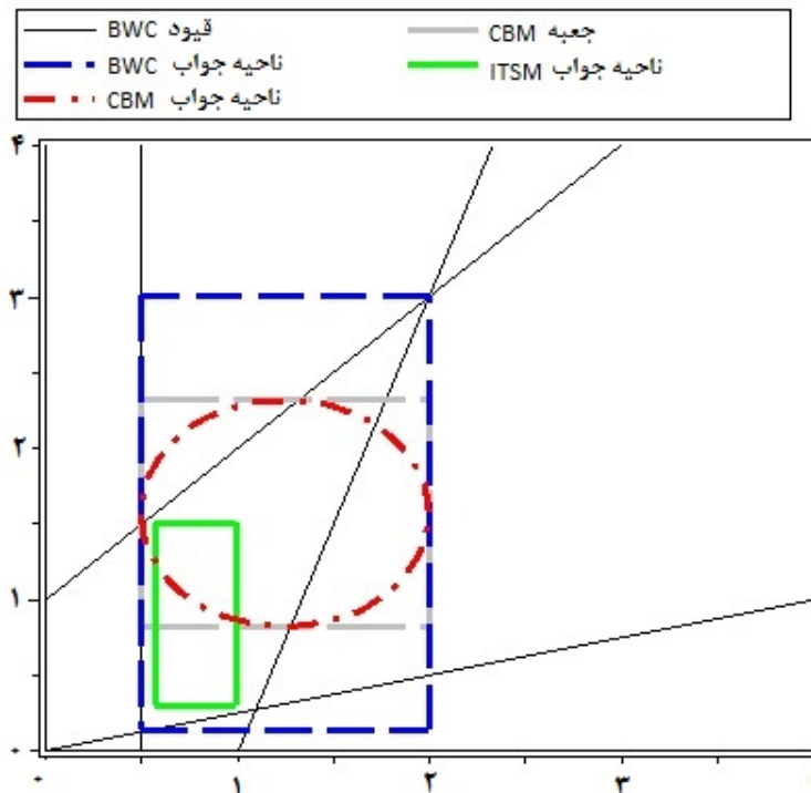
شکل ۲. نواحی جواب BWC، ITSM، CBM برای مدل (۶)
