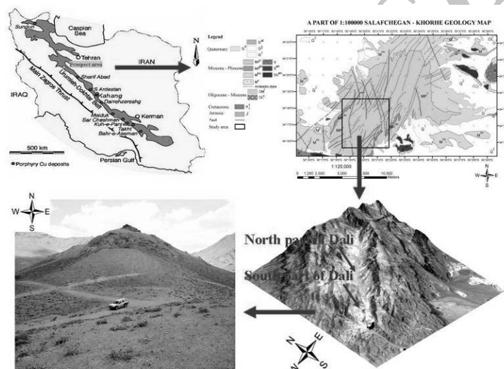
شکل ۱: موقعیت بخش‌های شمالی و جنوبی کانسار دالی بر روی نقشه زمین‌شناسی ۱:۱۰۰۰۰۰ سلفچگان- خورهره، تصویر سه‌بعدی داده‌های IKONOS و تصویر محدوده مورد مطالعه (دید به سمت شمال)
