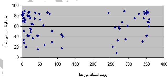
نمودار ۱: همبستگی بین جهت امتداد درزه‌ها و شیب درزه‌ها
