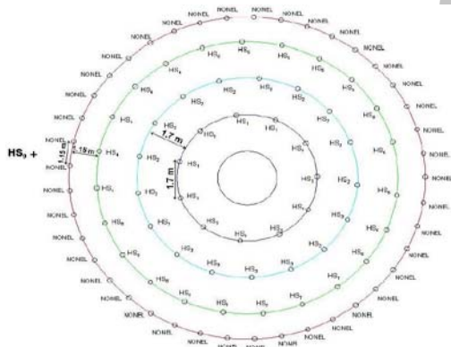
شکل ۲: الگوی پیشنهادی حفاری چال‌های انفجاری تمام‌مقطع
