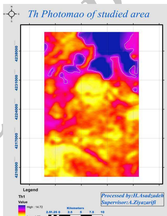
شکل ۴: نقشه کریجینگ شده داده‌های پتاسیم منطقه اکتشافی
