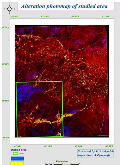
شکل ۱۰: استخراج آلتراسیون ها با روش تقسیم باندهای
