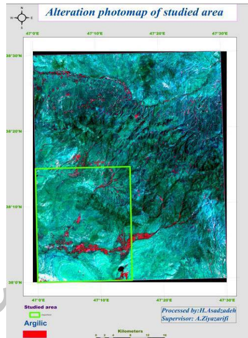
شکل ۹: استخراج آلتراسیون، با روش ترکیب باندهای
