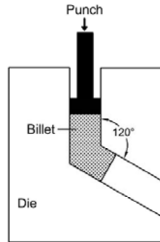
شکل ۱- طرح شماتیکی از کانالهای قالب.
