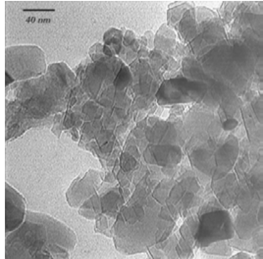
شکل ۳- تصاویر حاصل از آزمون میکروسکوپی الکترونی عبوری فورستريت در دو بزرگنمایی مختلف.
