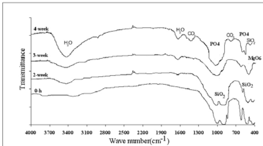
شکل ۴- طیف حاصل از طیف سنجی مادون قرمز نانوپودر فورستريت بعد از زمانهای ۰-۲۸ روز غوطه وری در محلول شبیه‌سازی شده بدن.
