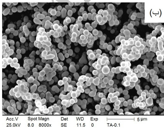
شکل ۴- نمونه سنتز شده با نسبت (الف) ۰/۱ مولی اتیلن گلیکول و (ب) ۰/۰۱ مولی نیترو بنزن
