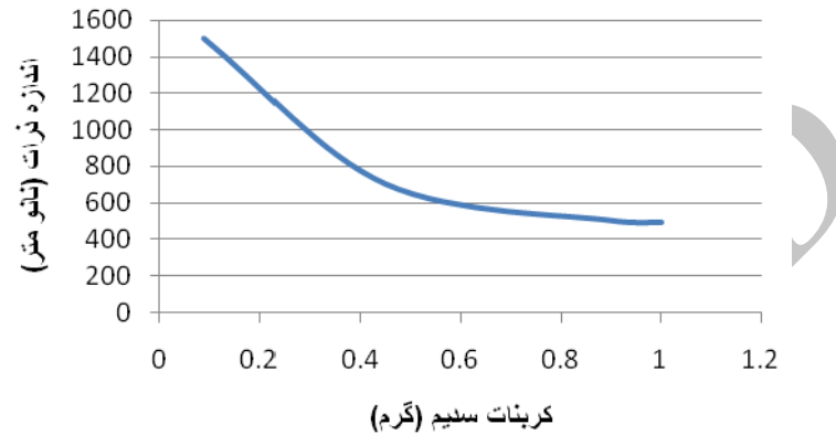
شکل ۳- نمودار تأثیر افزودن مقادیر مختلف کربنات سدیم بر اندازه و همسانی ذرات
