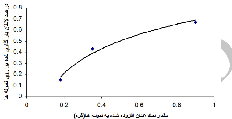
شکل ۵- رابطه مقدار نمک اضافه شده به محیط واکنش با درصد وزنی نمک بارگذاری شده بر روی نمونه‌های سنتز شده
