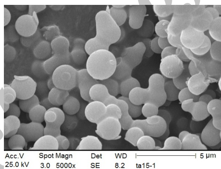
شکل ۶- نمونه سنتز شده به همراه ۰/۱۸ گرم لاتانیوم و ۳۰ دقیقه امواج اولتراسونیک
