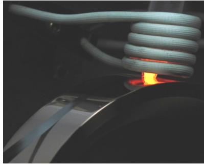
شکل ۱- طرح شمایی و تصویر فرایند ریخته ریسی [۴].
