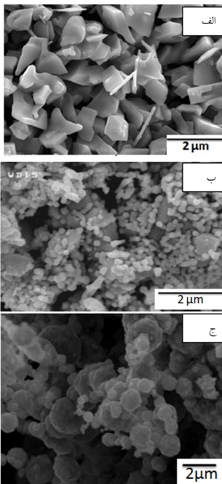
شکل ۱- تصاویر SEM (الف) پودر میکرو مولیبدن، (ب) نانو پودر مولیبدن و (ج) پودر نیکل
