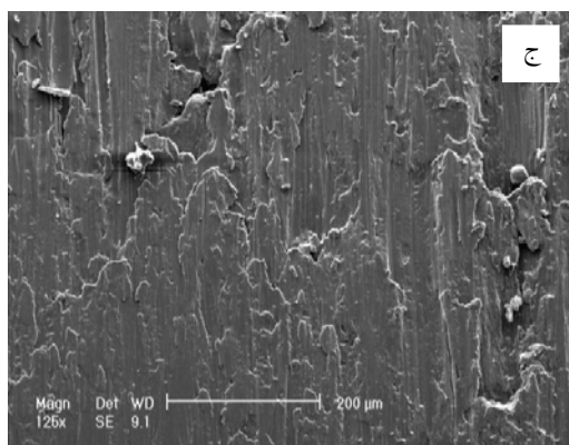
شکل ۱۴- تصویر میکروسکوپی الکترونی از سطوح سایشی نمونه‌ی ریختگی آلیاژ آلومینیم- ۱۱/۲٪ سیلیسیم،، (الف) قالب فلزی، فاقد جریان الکتریکی، (ب) قالب فلزی متصل شده به جریان الکتریکی متناوب و (ج) قالب فلزی متصل شده به قطب مثبت جریان الکتریکی مستقیم
