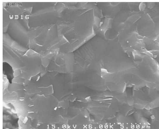
شکل ۱۰- تصویر ریزساختار ترکیب حاوی ۶ درصد افزودنی کلرید منیزیم پخته شده در دمای ۱۵۰۰ °C
