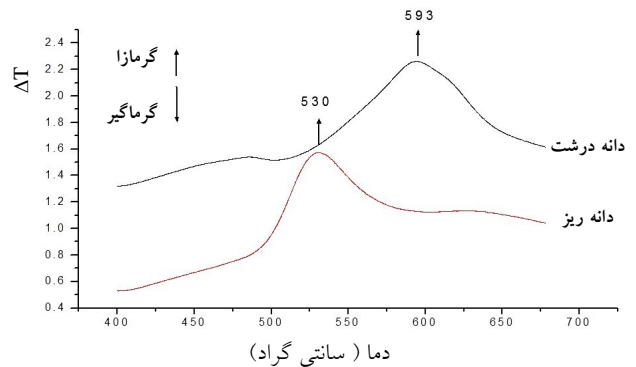
شکل ۴- آنالیز DTA شیشه حاوی جوانه زا در دو دانه بندی
