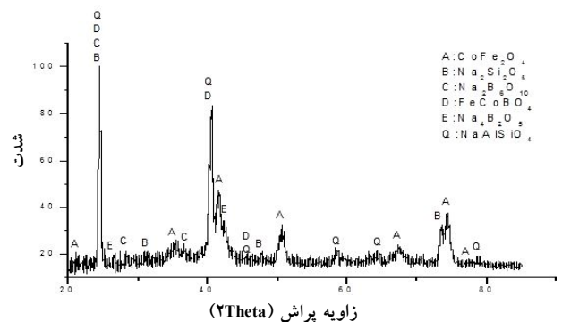
شکل ۶- الگوی XRD نمونه عملیات حرارتی شده در
