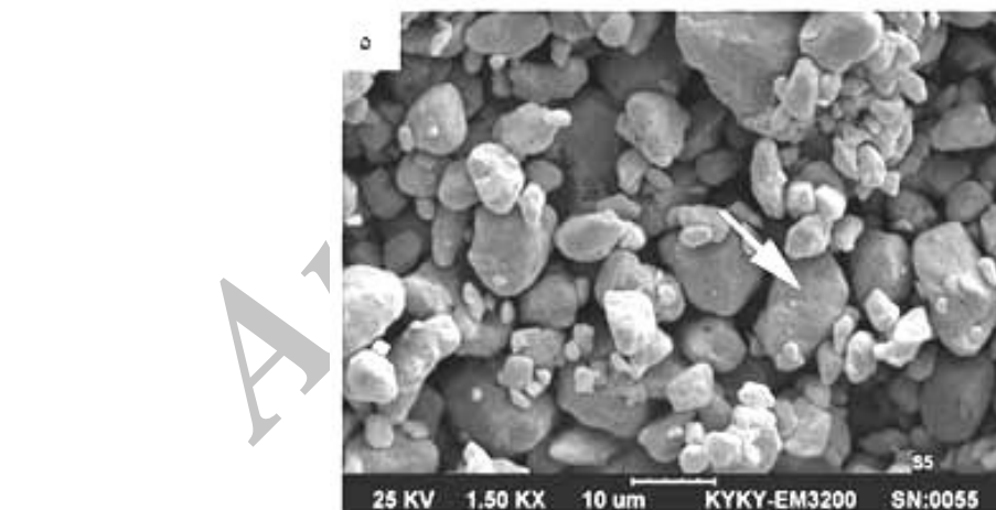
شکل ۱- تصاویر میکروسکوپ الکترونی روبشی از تغییر ریخت مخلوط پودری در زمان‌های مختلف آسیاب:
