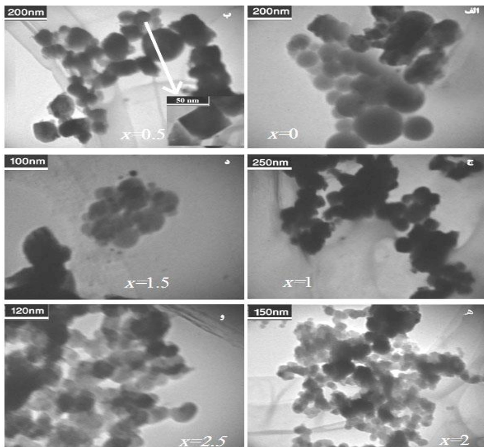
شکل ۷- تصاویر میکروسکوپی الکترونی عبوری نانو ذرات فریت استرانسیم با ترکیب شیمیایی \text{SrFe}_{12-2x}(\text{MgCo})_{0.5x}\text{Ti}_x\text{O}_{19} (به ازاء الف) x=0 ، (ب) x=0.5 ، (ج) x=1 ، (د) x=1.5 ، (ه) x=2 و (و) x=2.5
