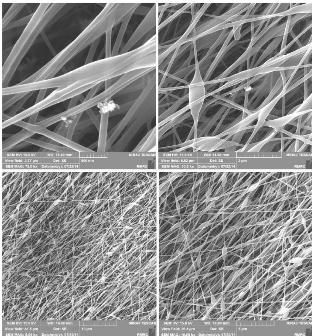
شکل ۴- تصاویر میکروسکوپ الکترونی گسیل میدانی از نمونه داربست نانوکامپوزیتی الکترورسی شده کیتوسان/ پلی وینیل الکل/ نانولوله کربنی/ شیشه زیست فعال اتصال عرضی شده در بزرگ‌نمایی‌های مختلف
