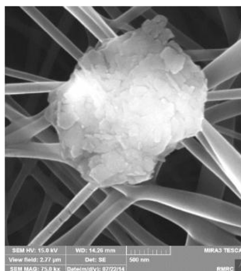
شکل ۳- تصاویر میکروسکوپ الکترونی گسیل میدانی از نمونه داربست نانوکامپوزیتی الکتروزی شده کیتوسان/ پلی وینیل الکل / نانولوله کربنی / شیشه زیست فعال اتصال عرضی نشده در بزرگنمایی های مختلف
