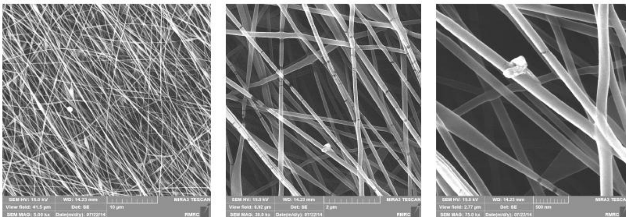
شکل ۱- تصاویر میکروسکوپ الکترونی گسیل میدانی از نمونه داربست نانوکامپوزیتی الکترورسی شده کیتوسان/ پلی وینیل الکل / نانولوله کربنی اتصال عرضی نشده در بزرگ‌نمایی‌های مختلف
