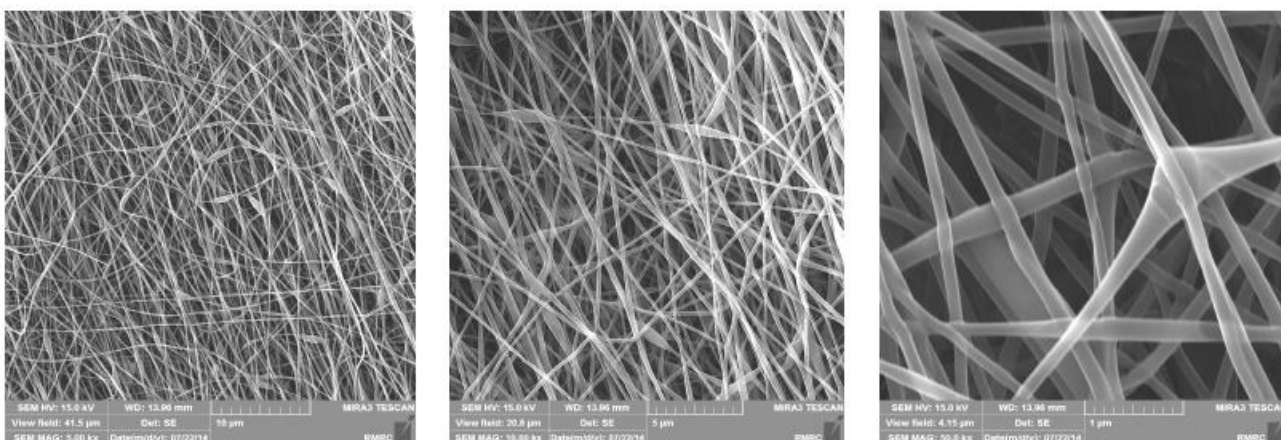
شکل ۲- تصاویر میکروسکوپ الکترونی گسیل میدانی از نمونه داربست نانوکامپوزیتی الکترورسی شده کیتوسان/ پلی وینیل الکل / نانولوله کربنی اتصال عرضی شده در بزرگ‌نمایی‌های مختلف
