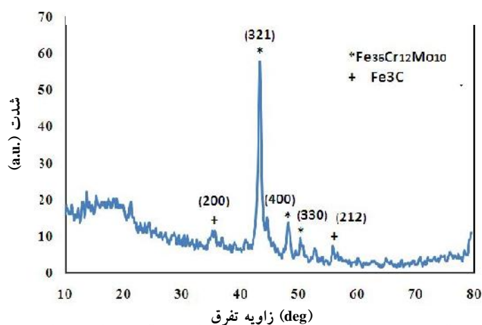
شکل ۱۲- منحنی تفرق اشعه ایکس آلیاژ Fe_{52}Cr_{18}Mo_7B_{16}C_4Nb_3 پس از انجام عملیات حرارتی در دمای 650^\circ درجه سانتی گراد به مدت زمان ۳ ساعت
