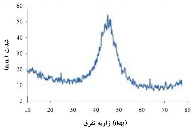
شکل ۱۰- منحنی تفرق اشعه ایکس آلیاژ Fe_{50}Cr_{18}Mo_7B_{16}C_4Nb_5 در حالت آمورف
