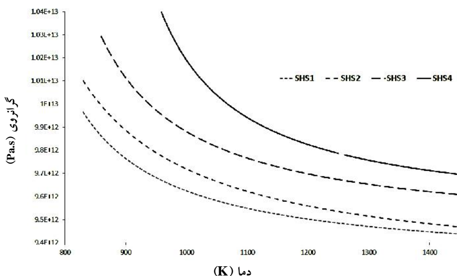
شکل ۲۷- منحنی تغییرات گرانی با دما برای آلیاژها
